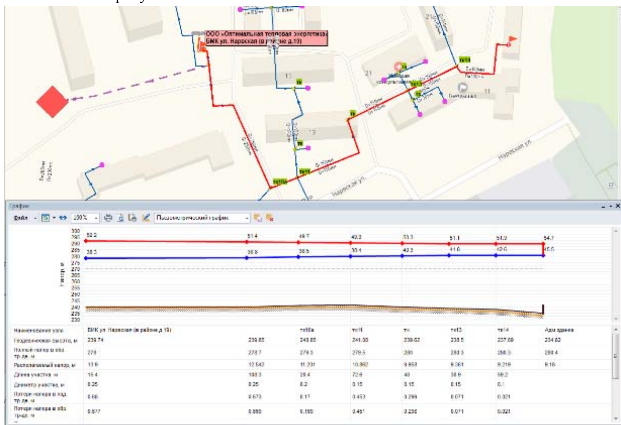
Рисунок 3.5 – Результат гидравлического расчета тепловых сетей
