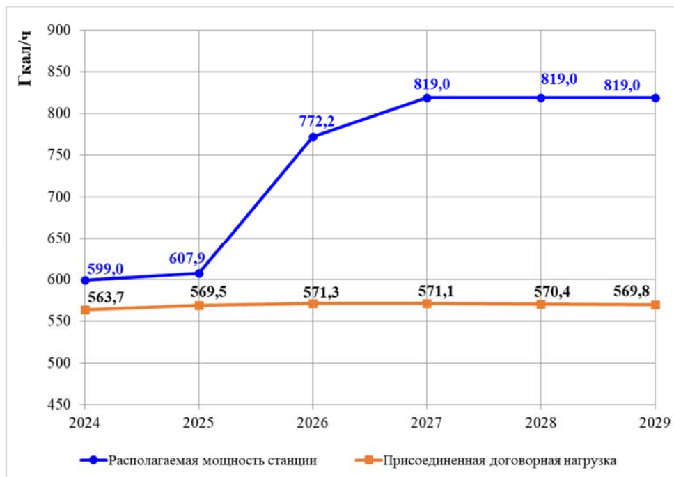
Рисунок 7.1 – График обеспеченности покрытия присоединенных тепловых нагрузок Смоленской ТЭЦ-2
