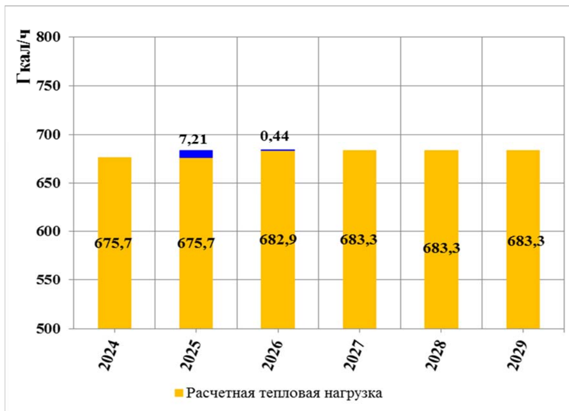
Рисунок 2.2 – Расчетная тепловая нагрузка и прирост тепловой нагрузки на расчетный период
