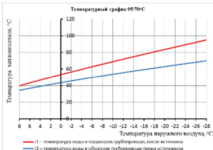
Рисунок 9.2 – Температурный график 95/70 °C котельных МУП "Смоленсктеплосеть" №№ 1, 2, 6, 7, 8, 12, 13, 16, 18, 19, 20, 23, 24, 25, 26, 28, 29, 32, 33, 35, 36, 37, 38, 40, 41, 44, 53, 54, 55, 66, 67, 69, котельной "Хладосервис", котельной ул. Кутузова
