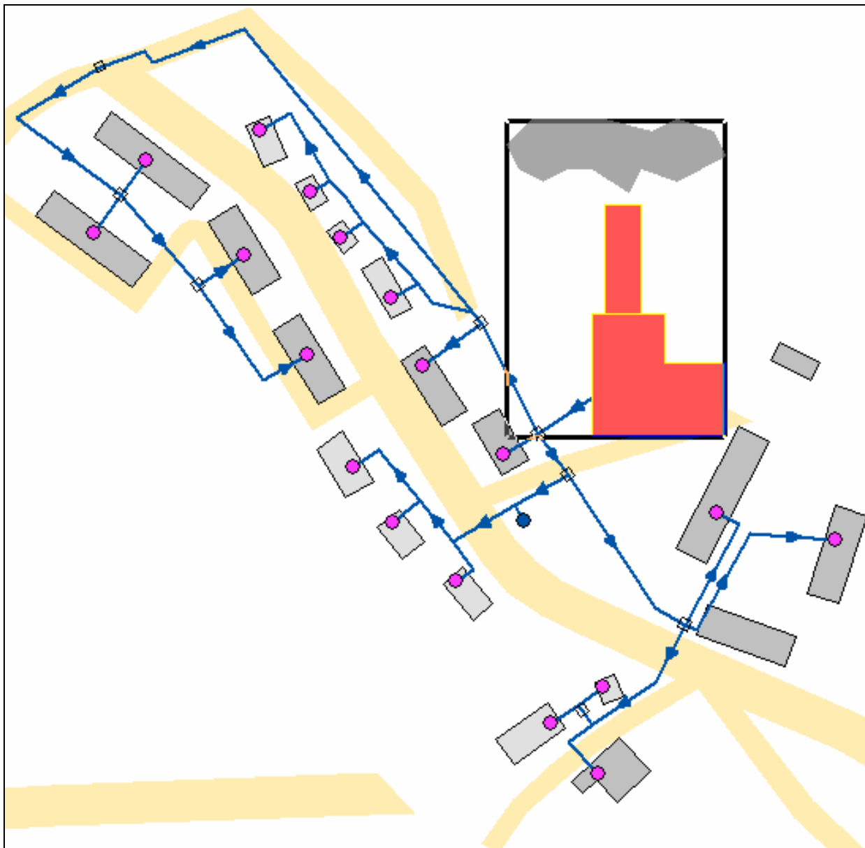
Рисунок Е 27– Схема тепловых сетей котельной № 37
