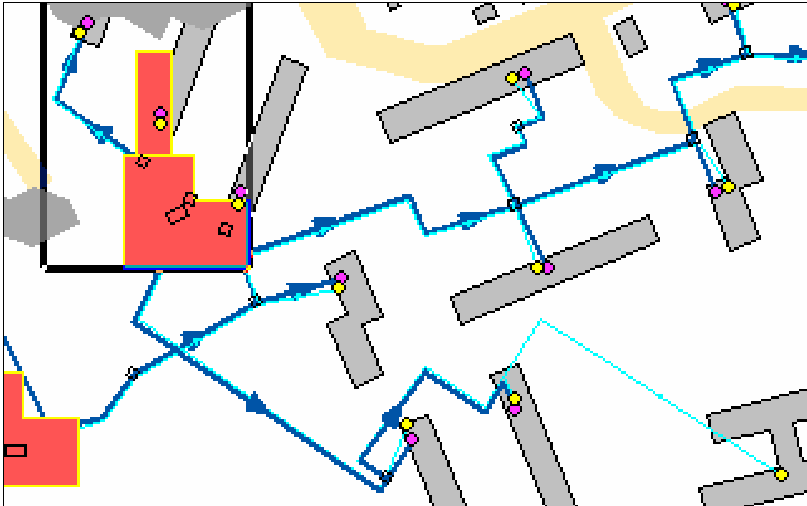
Рисунок Е 5– Схема тепловых сетей котельной № 6
