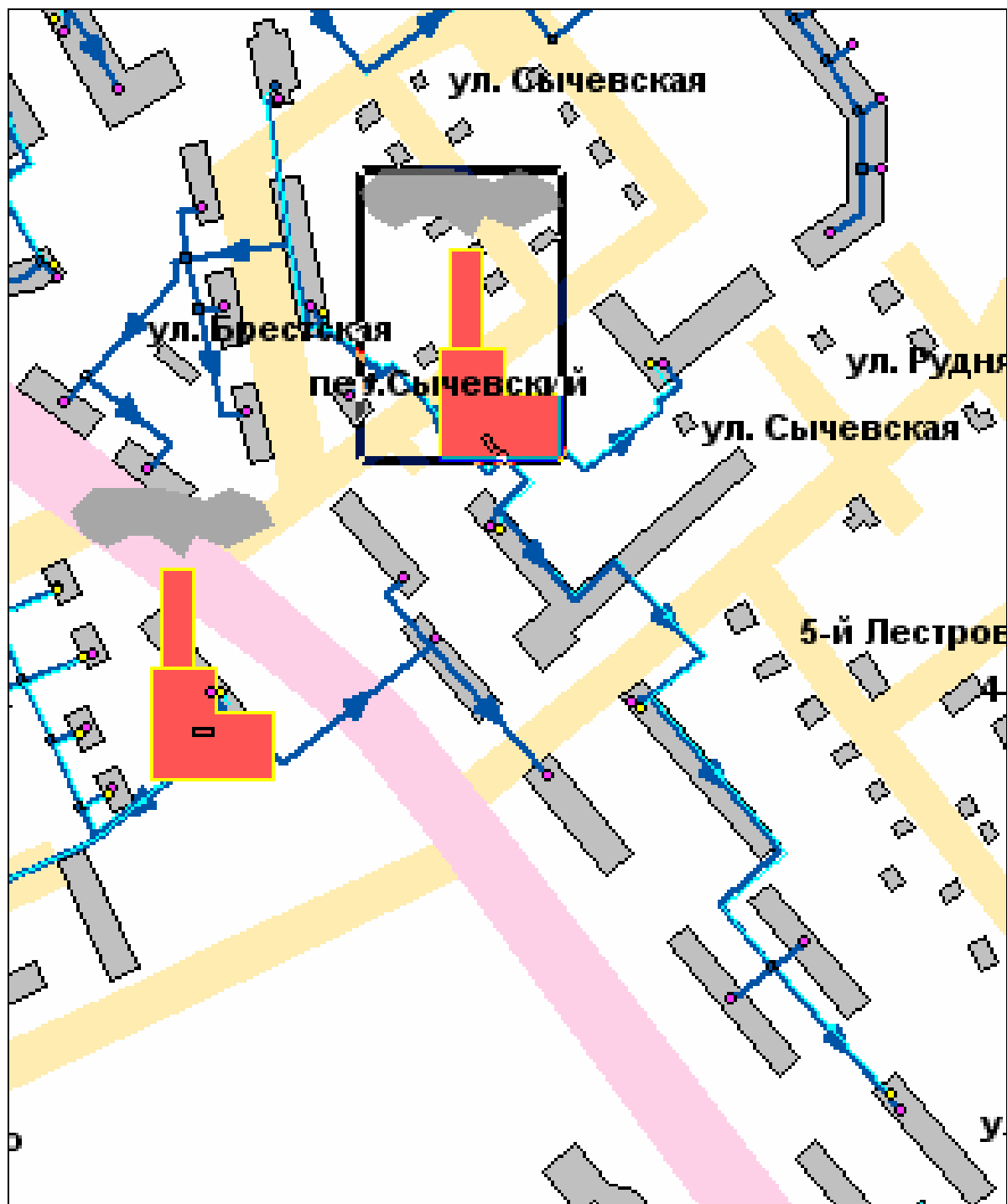
Рисунок Е 26– Схема тепловых сетей котельной № 36
