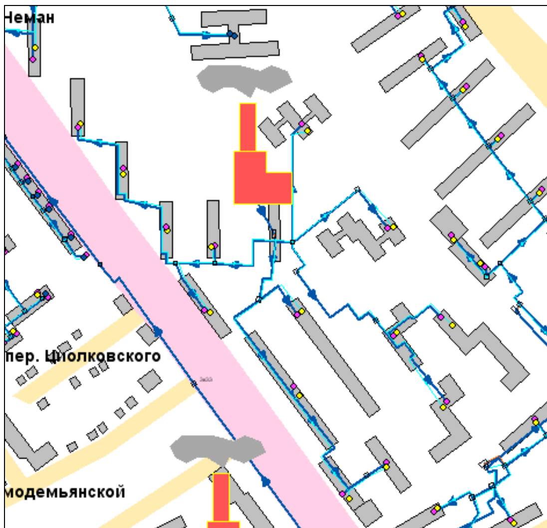
Рисунок Е 1 – Схема тепловых сетей котельной № 1
