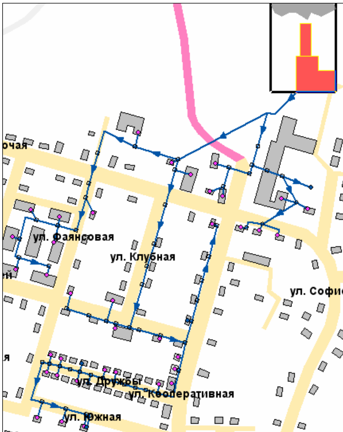
Рисунок Е 23– Схема тепловых сетей котельной № 33
