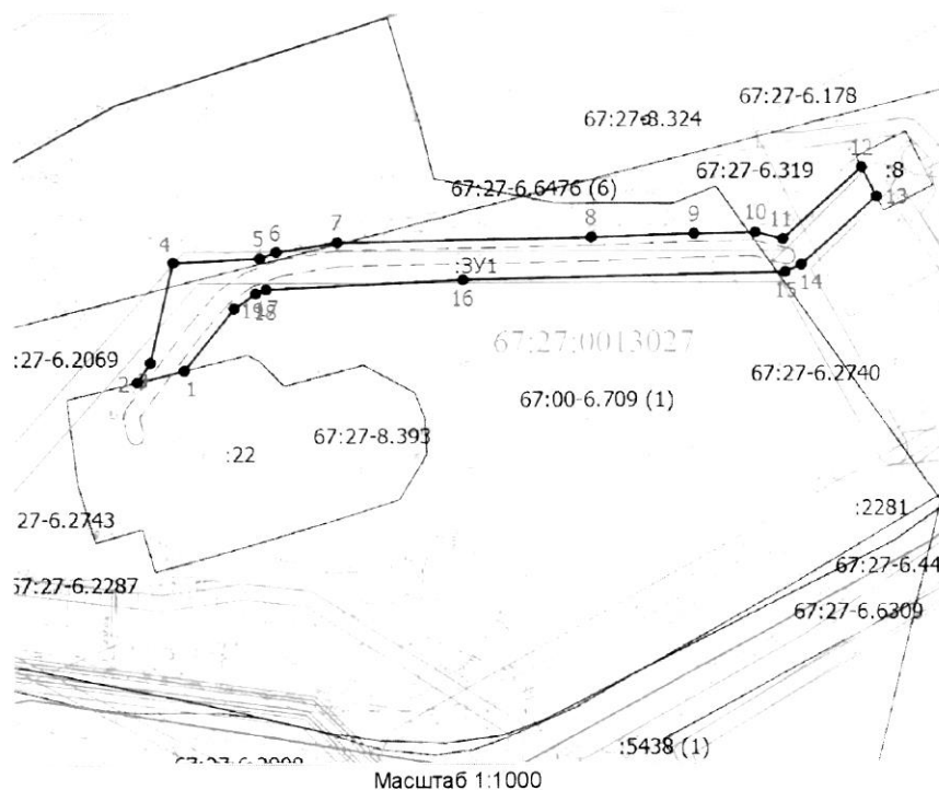
ЧЕРТЁЖ РАЗМЕЩЕНИЯ ОБЪЕКТА на предполагаемых к использованию землях
