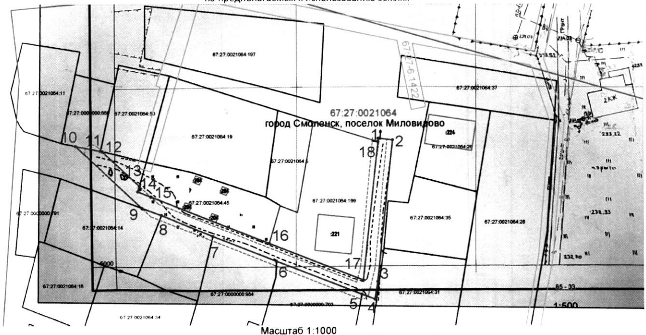
ЧЕРТЕЖ РАЗМЕЩЕНИЯ ОБЪЕКТА на предполагаемых к использованию землях
