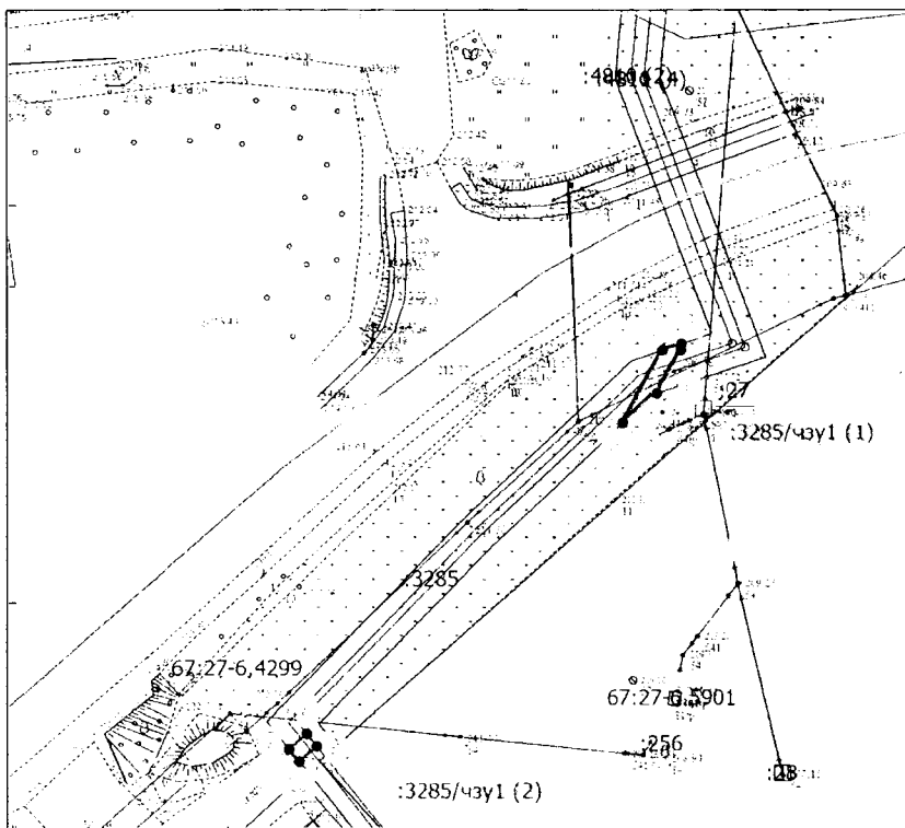
ЧЕРТЁЖ РАЗМЕЩЕНИЯ ОБЪЕКТА на предполагаемых к использованию землях
